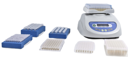
MPS-1 高速微量盤旋轉震盪器
